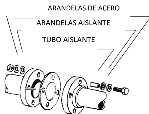
JUNTA DIELECTRICA TIPO E
